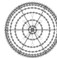
Top View(1:2)
